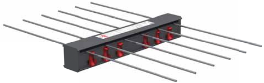
HIT-MVX für Auskragende Balkone
